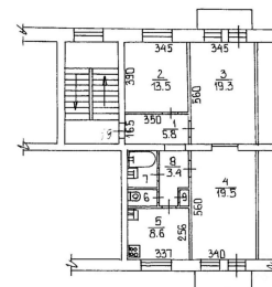
ПЛАН КВАРТИРЫ № 19 (выкопировка из поэтажного плана дома) М1:200
