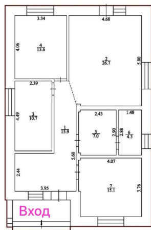
1-й ЭТАЖ
