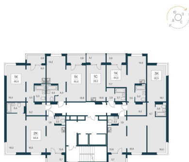
ПЛАН 2-17 ЭТАЖА
